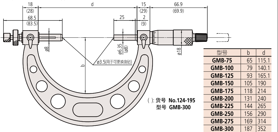
测量范围 50mm-300mm 普通型 GMB-75 ~ 300
