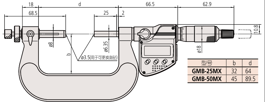
测量范围 50mm-100mm 数显型 GMB-75MX ~ 100MX
