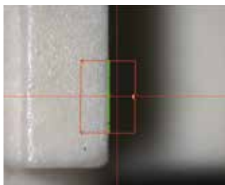
用环形照明的左侧进行照射，突出边缘以进行测量
